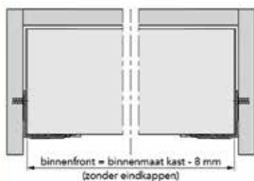
Front voor Vionaro binnenlade met hoogte 121 mm
